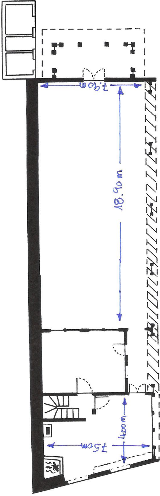
Erdgeschoss
